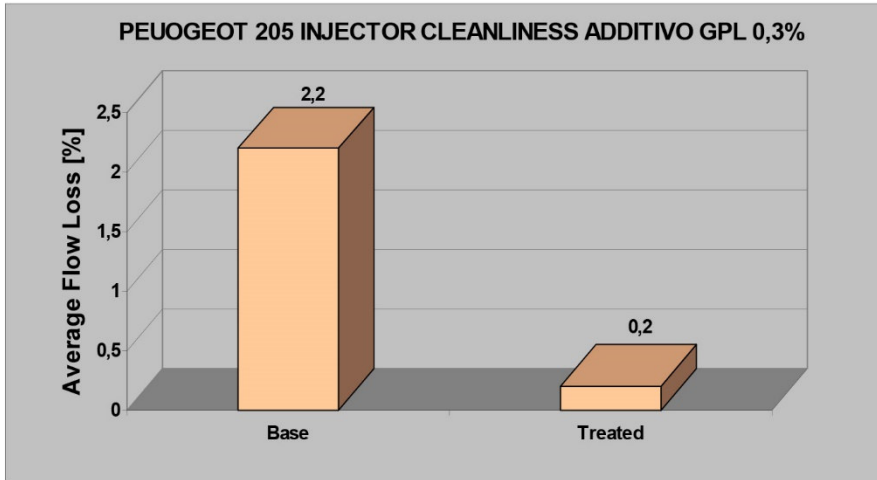
Grafico 3: benefici nell'utilizzo di PULITORE GPL in relazione alla perdita di flusso in spirazione
