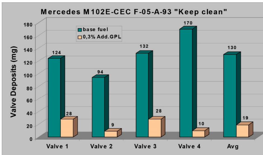
Grafico 4: benefici nell'utilizzo di PULITORE GPL in relazione ai depositi sulle valvole
