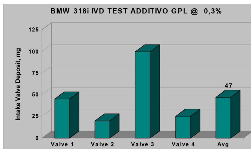
Grafico 2: benefici nell'utilizzo di PULITORE GPL in relazione ai depositi sulla valvola di aspirazione
