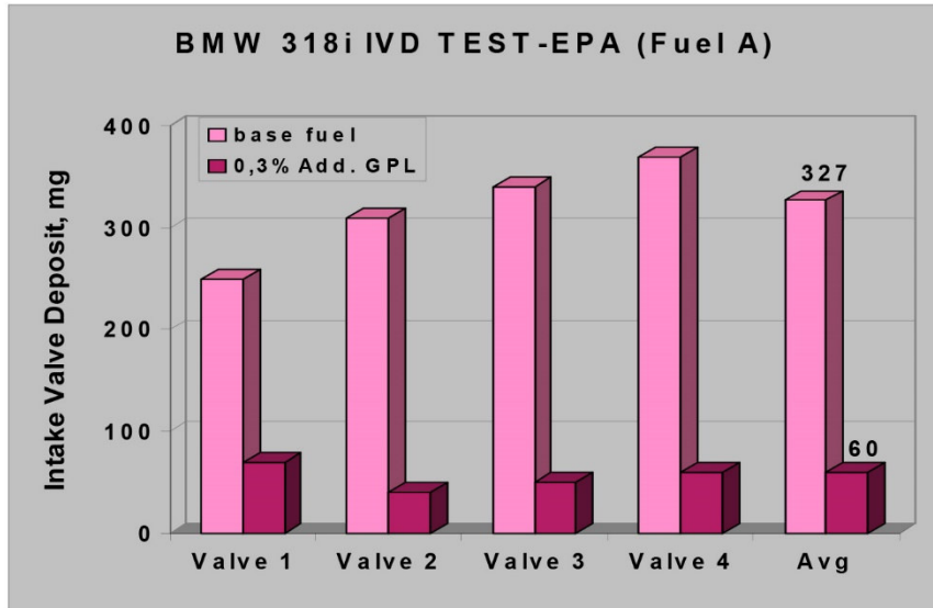
Grafico 6: benefici nell'utilizzo di PULITORE GPL in relazione ai depositi sulle valvole
